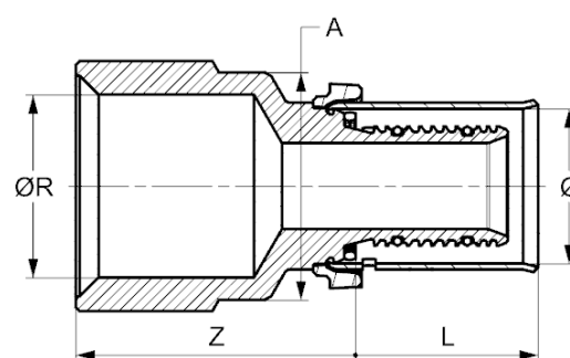
Vue en coupe avec cote
