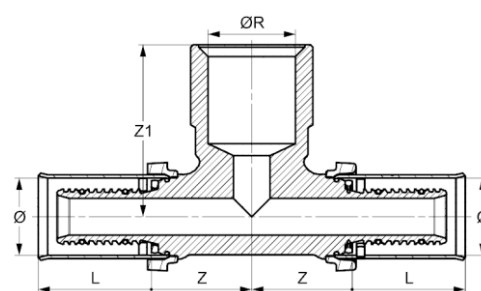
Vue en coupe avec cote
