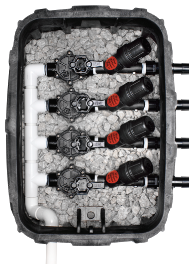
Quatre kits de départ dans un regard de vanne traditionnel
